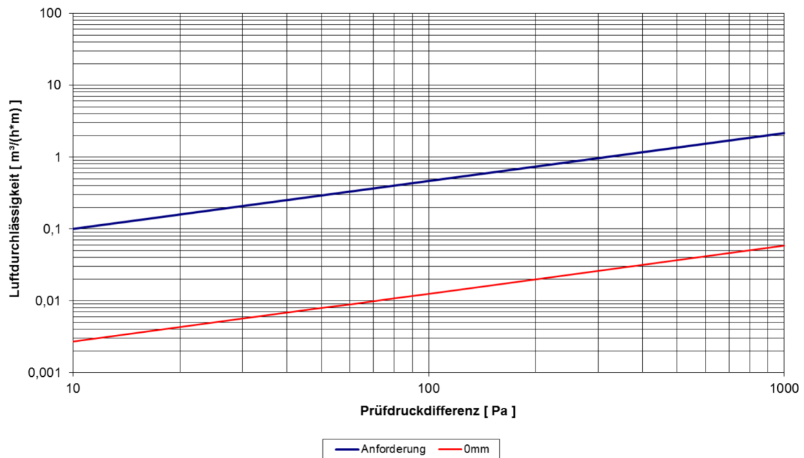
Abbildung 4: Luftdurchlässigkeit (M120)
